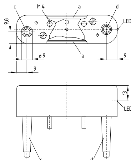
Cable outlet
