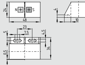
BP 20 N / BP 20 S
