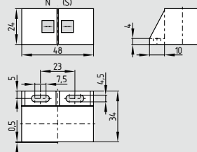
BP 31 N / BP 31 S
