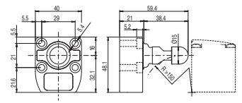
Actuator VN NG-F3•
