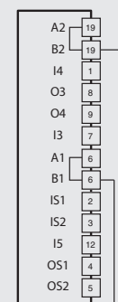
NG 2D••~•1G-K601 NG 2D••~•1H-K601 NG 2D••~•3G-K601
