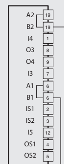
NG 2D••~•1E-K602 NG 2D••~•1F-K602 NG 2D••~•7F-K602
