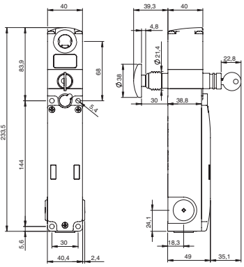
Actuator VN NG-F3•
