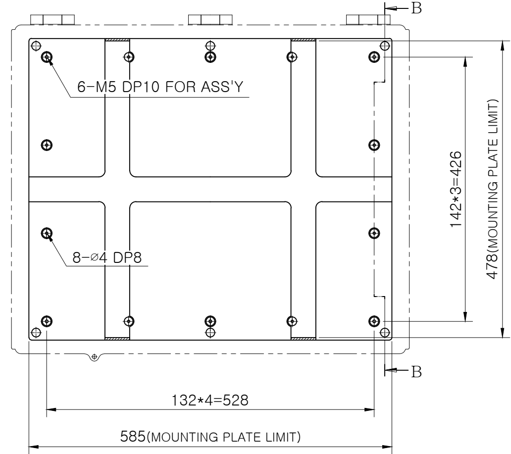
SECTION A-A
