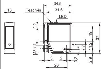
Masszeichnung OM30 Dimensional drawing OM30 Plan coté OM30
