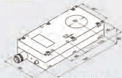
KJR-D50FAN-DNA-V2 KJR-D50FAN-DPA-V2
