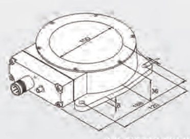
KJR-D100FAN-DNA-V2 KJR-D100FAN-DPA-V2
